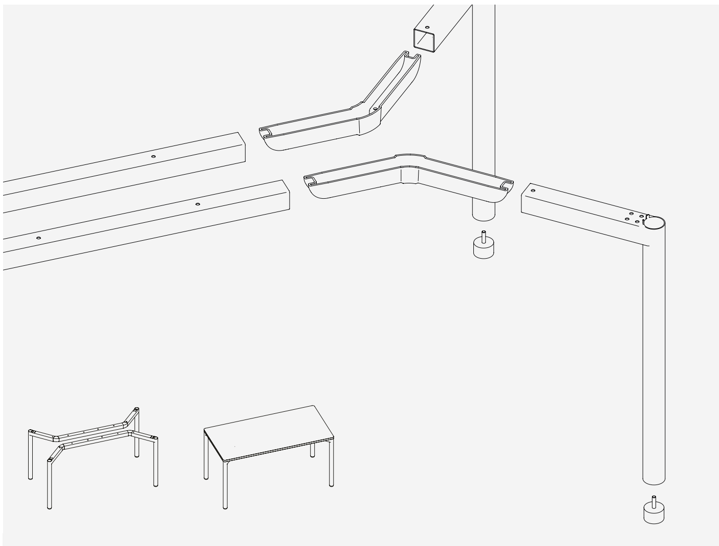
L-Verbindungselemente / L-connector
