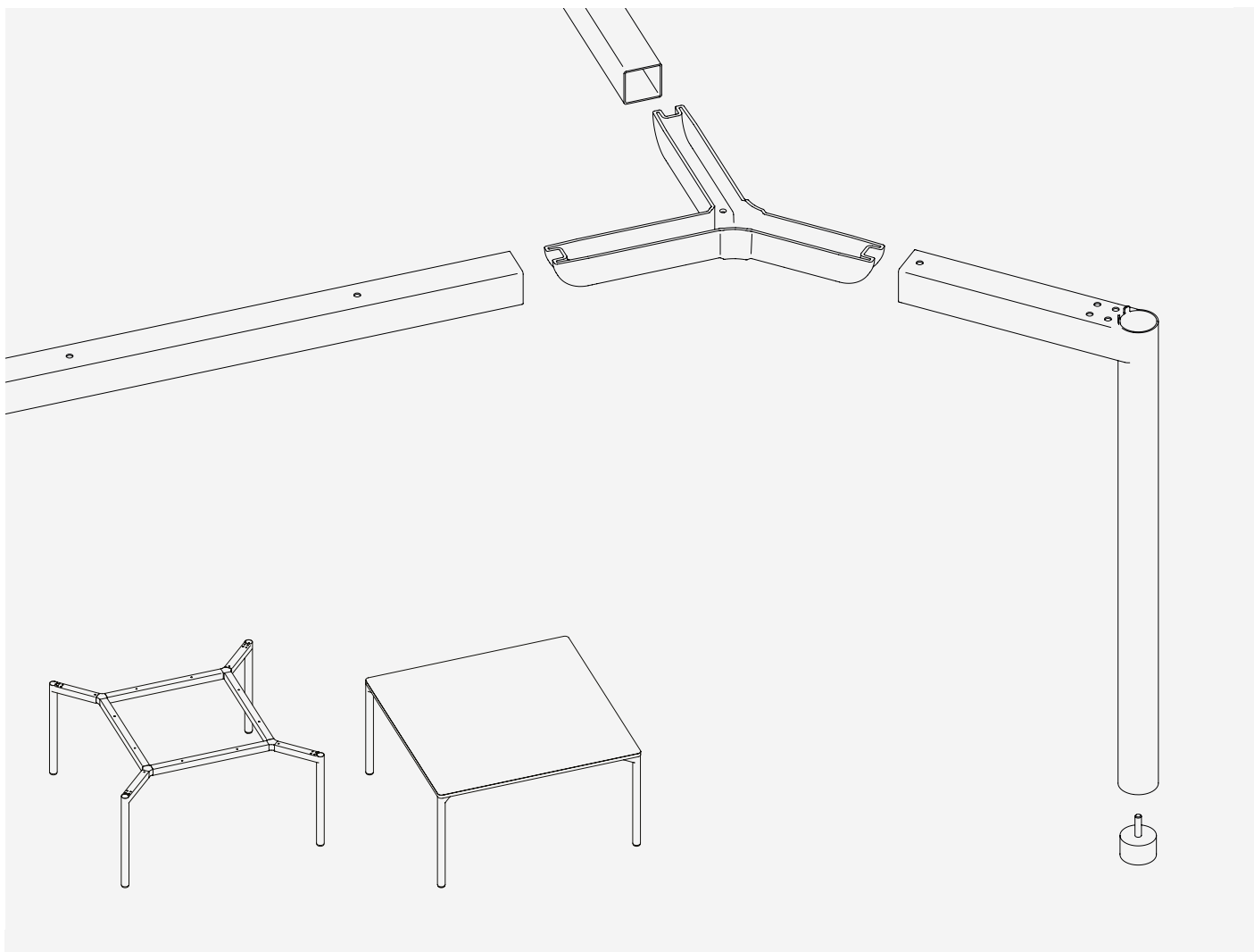
Y-Verbindungselemente / Y-connector
